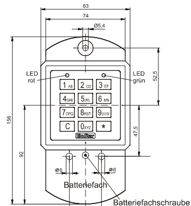
Tastatur 7231 senkrecht Batteriefach unten
