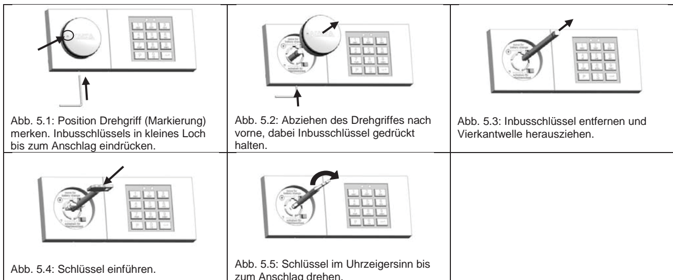
Abbildung 5: Schlüsselöffnung
