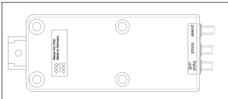
Abbildung 3: Schlossgehäuse
